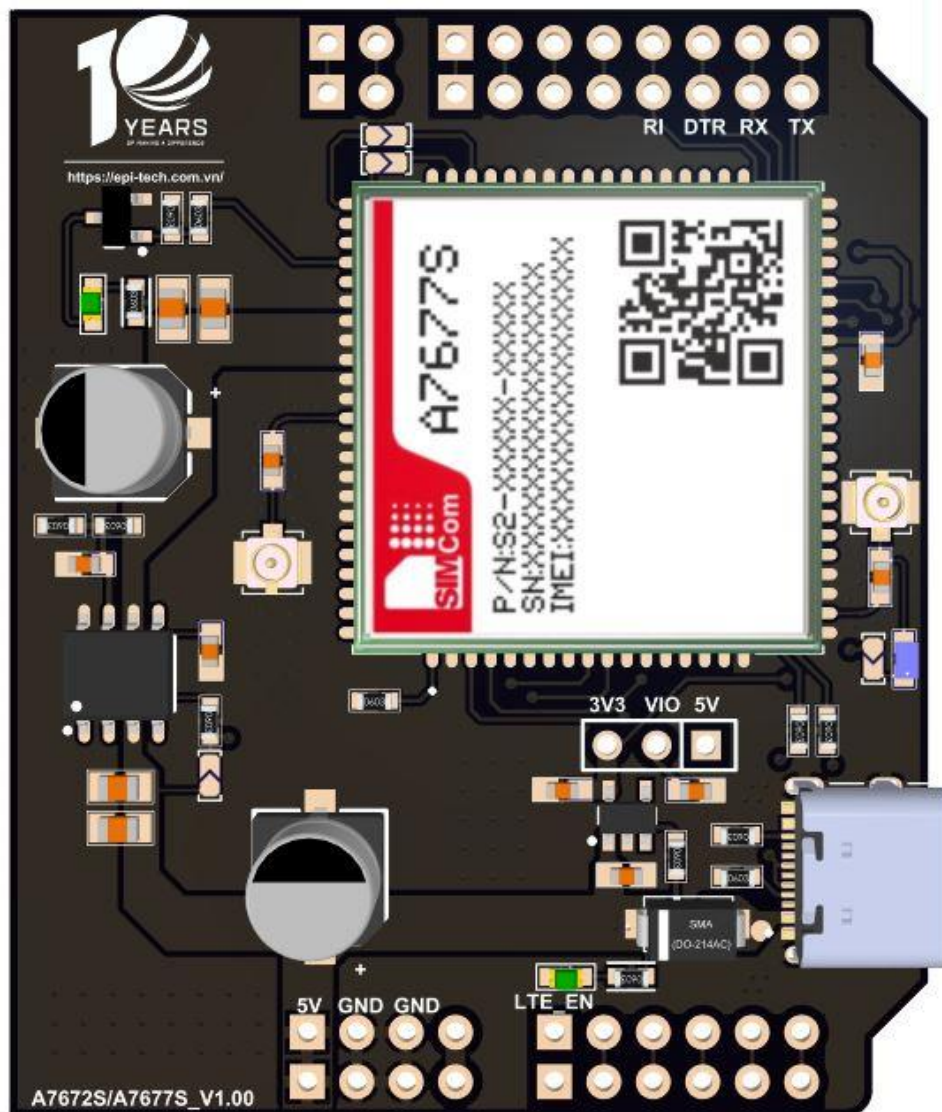
SIMCom A7677 Arduino Shield
